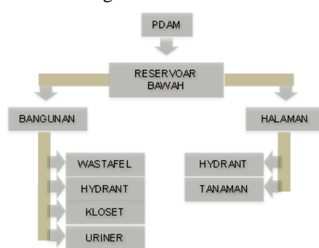
Gambar 4. Jaringan Air Bersih Sumber : Analisis, 2019
