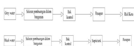
Gambar 5. Jaringan Air Kotor Sumber : Analisis, 2019
