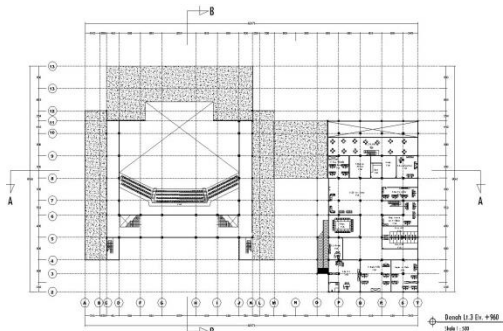
Gambar 13. Denah Lantai Elevasi +960
