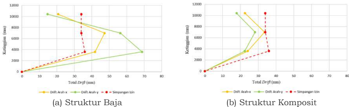
Gambar 4. Simpangan Antar Lantai Pada Struktur
