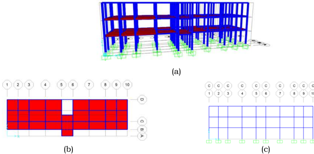
Gambar 1. Pemodelan Struktur
